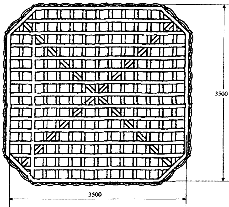
Конструкция ПСН
